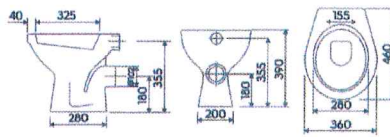
Technische Zeichnung
